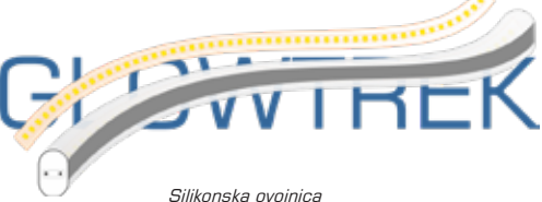
Silikonska ovojnica Presjek cijevi, 15mm x 8mm
